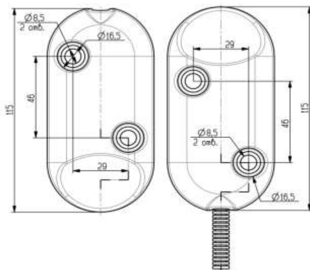
рис.1. Габаритные и установочные размеры. Высота задающего и исполнительного блока – 14 мм.
