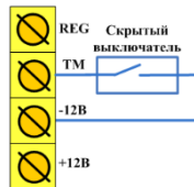
Рисунок 6.5 — Схема подключения скрытого выключателя или кнопки
