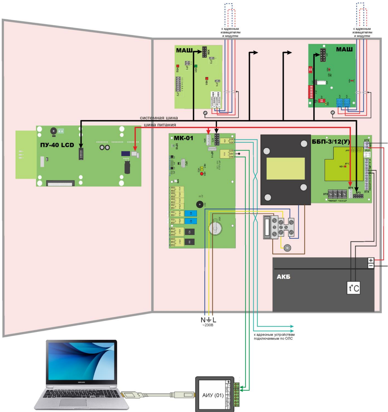
Рисунок 13. Схема подключения ППКиУ при инсталляции.
