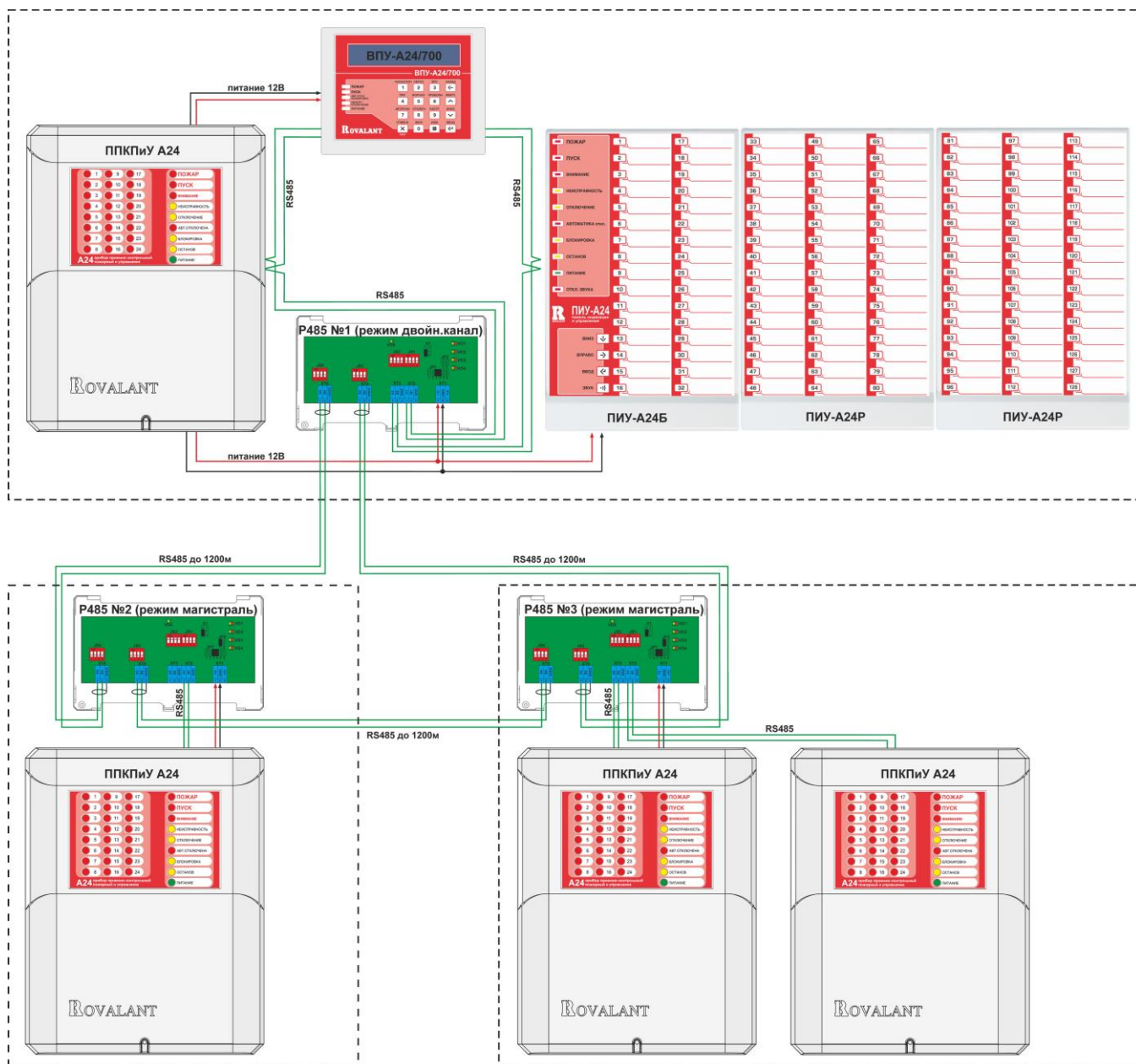
Рисунок 75. Схема подключения R485 для организации кольцевой гальвано-развязанной линии связи с сегментированной защитой от коротких замыканий.
