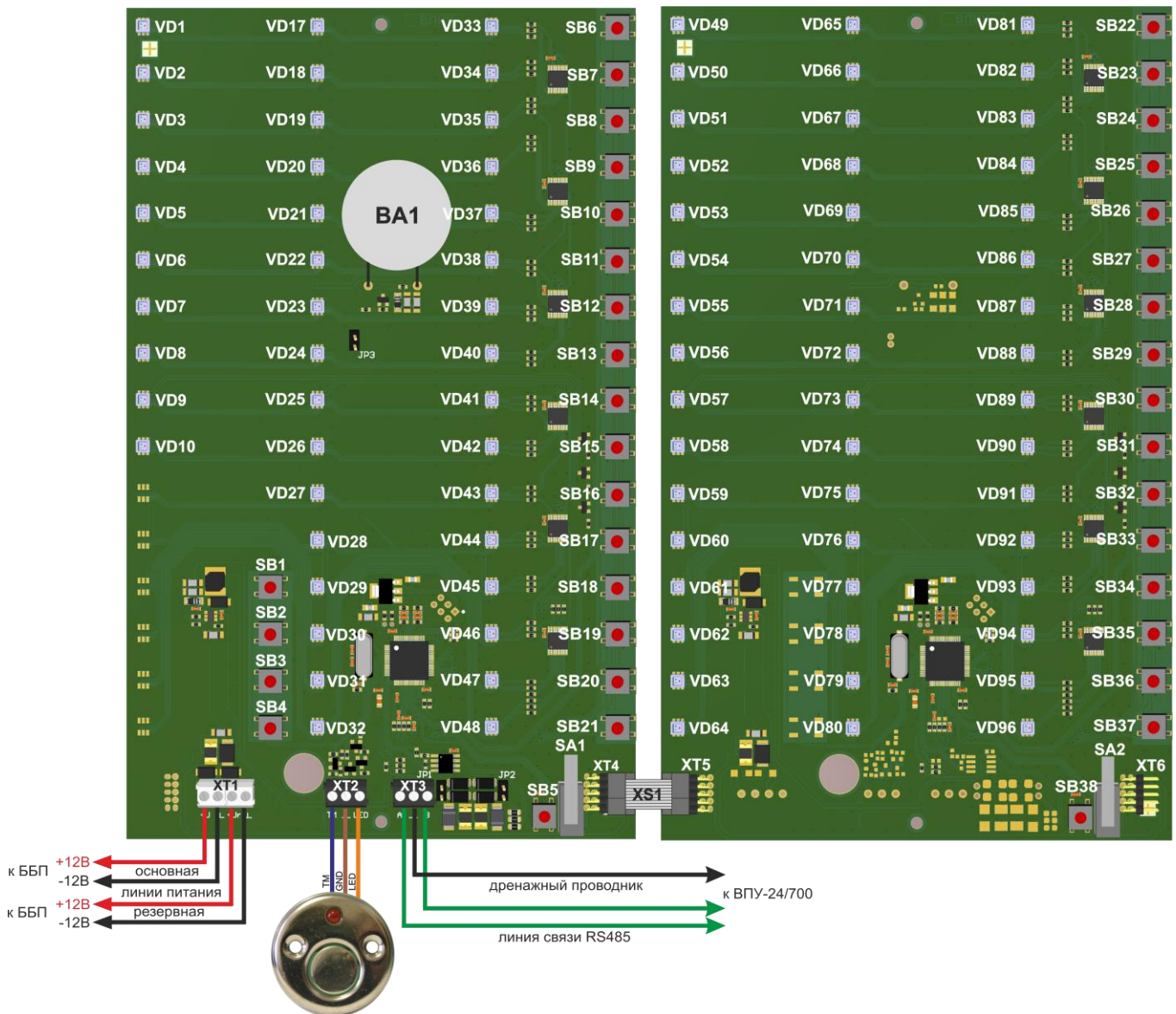
Рисунок 71 Внешний вид и подключение плат ПИУ-A24A
