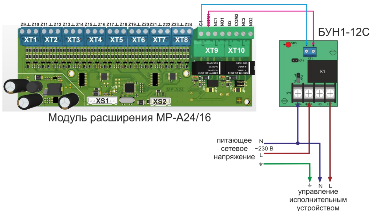
Рисунок 78. Схема подключения БУН1-12С к МР-А24/16.
