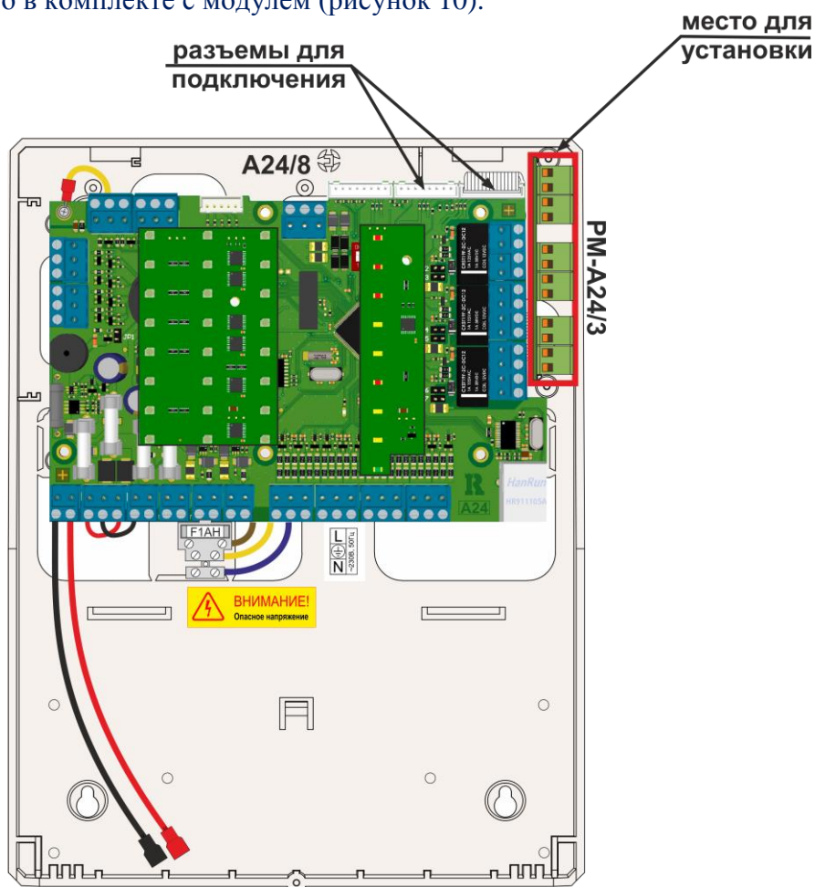
Рисунок 10. Установка РМ-А24/3 в корпус А24
