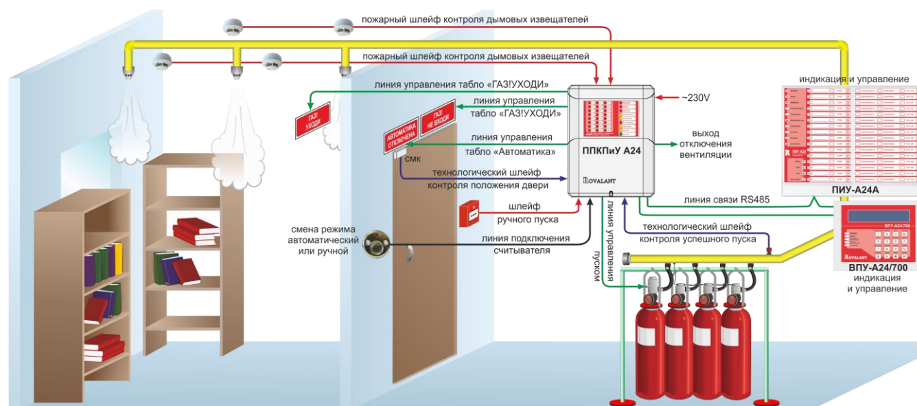
Рисунок 96. Пример автоматизации системы модульного газового АПТ
