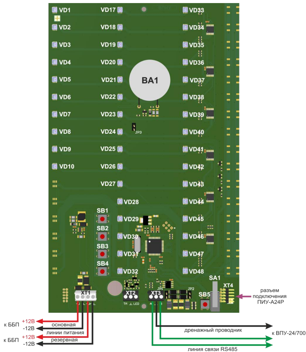
Рисунок 66. Внешний вид и подключение платы ПИУ-A24Б
