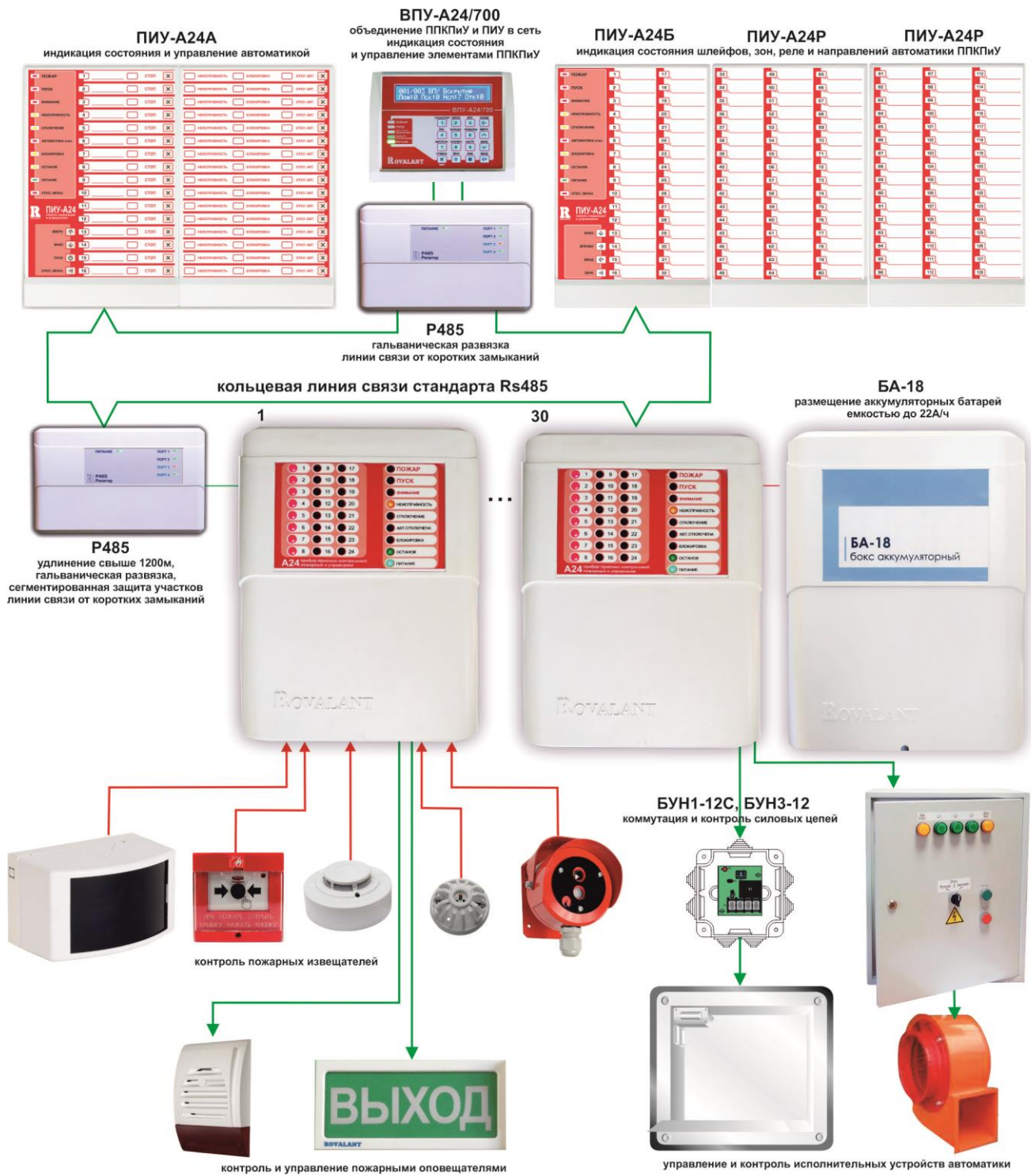
Рисунок 1. Структурная схема объединения ППКПиУ и компонентов
