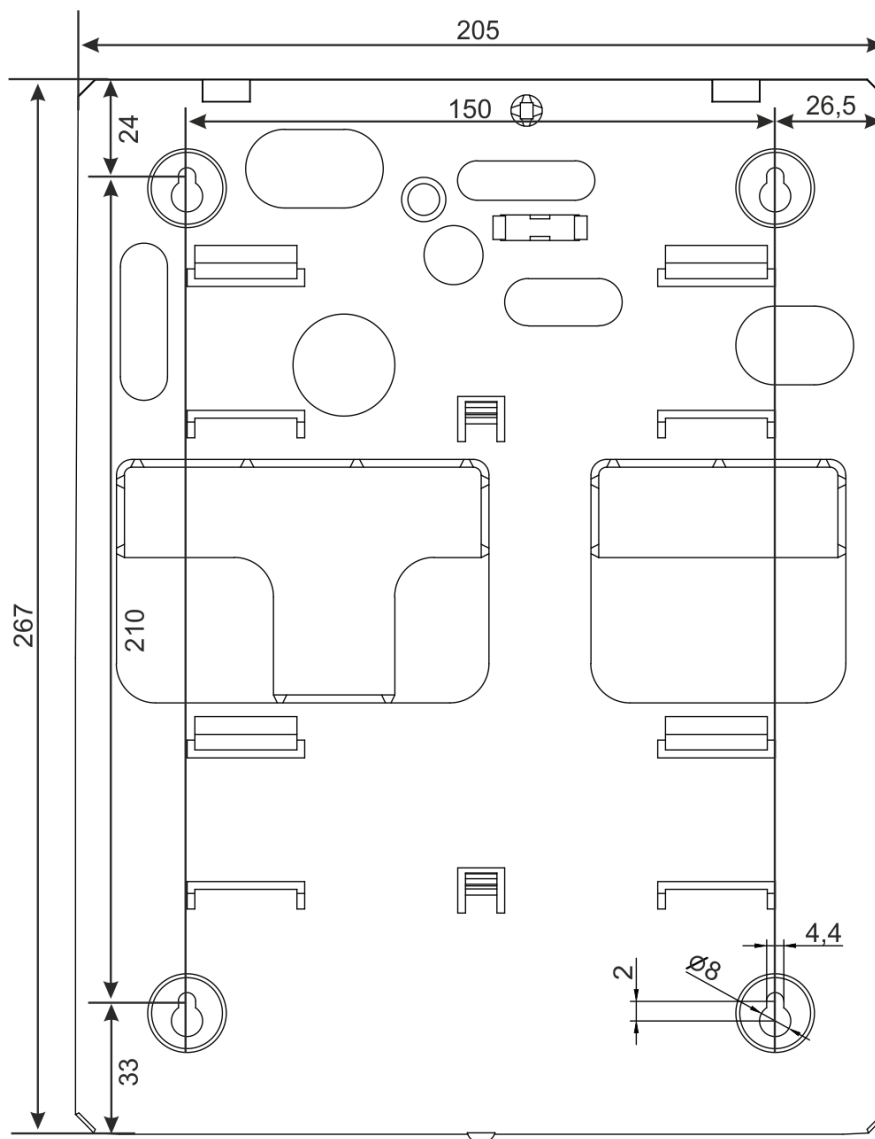
Рисунок 85. Установочный чертеж основания корпуса ППКПиУ серии «А24» и бокса аккумуляторного БА-18
