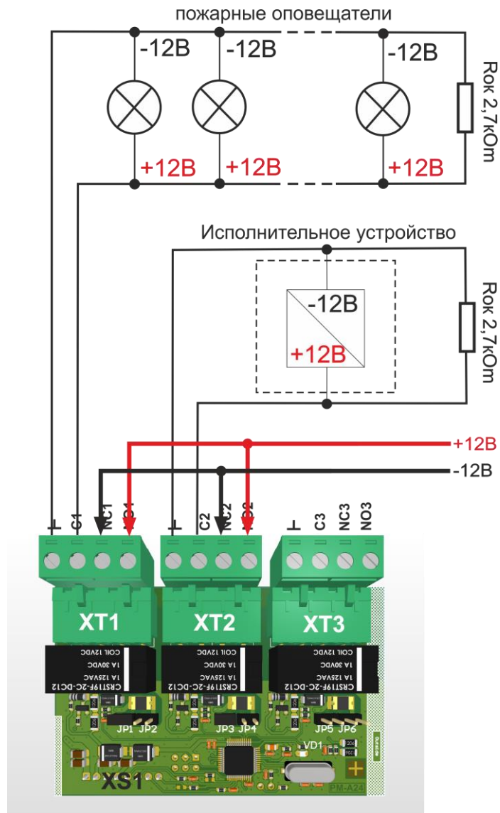
Рисунок 12. Схема подключения РМ-А24/3
