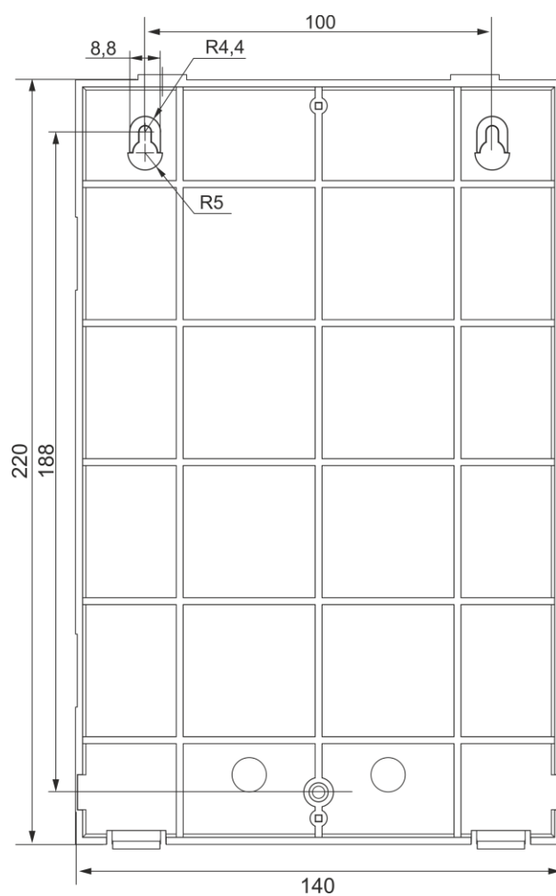
Рисунок 87. Установочный чертеж основания корпуса ПИУ-А24Б
