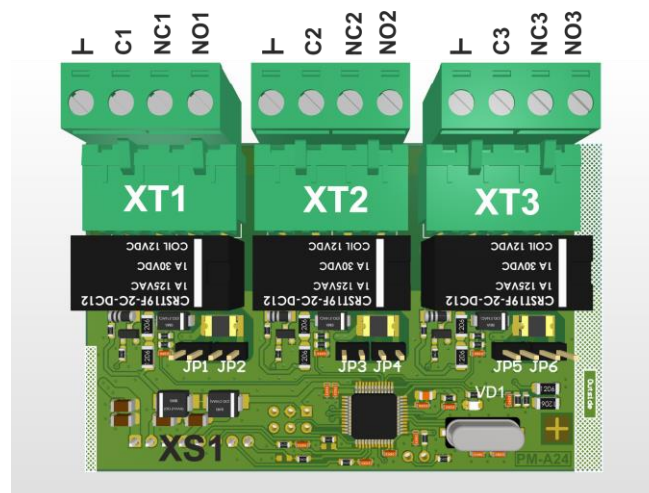
Рисунок 11. Внешний вид и обозначение элементов РМ-А24/3
