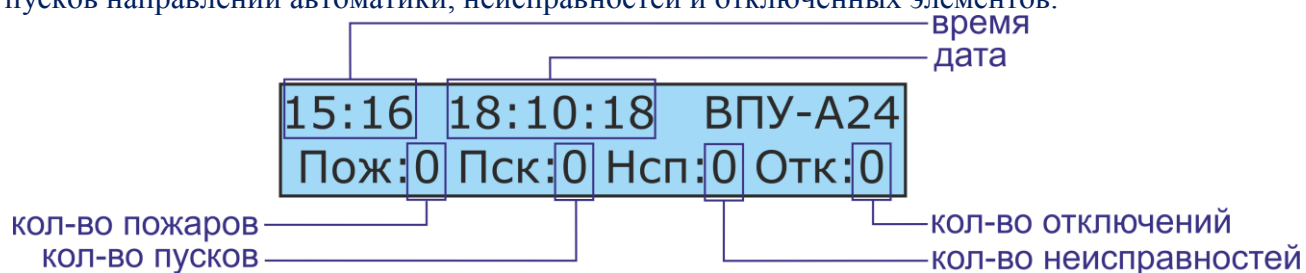
Рисунок 16. Индикация дисплея в дежурном режиме
