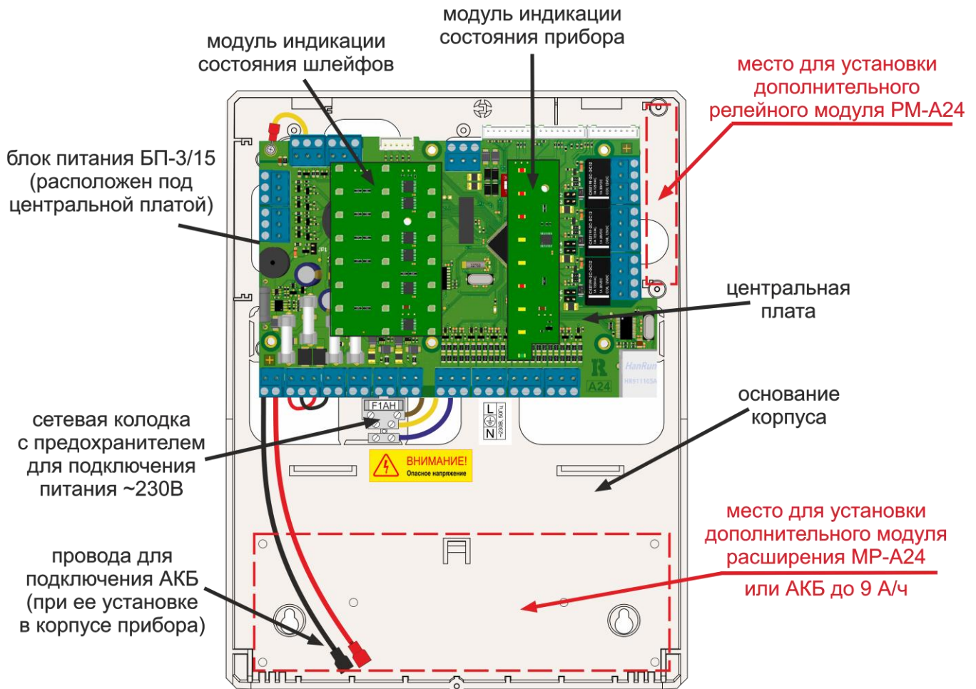
Рисунок 3. ППКПиУ с открытой передней крышкой.
