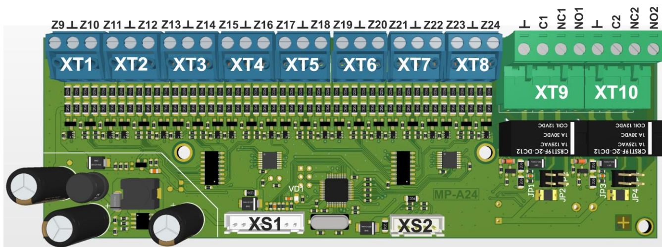
Рисунок 8. Внешний вид и обозначение элементов MP-A24/16
