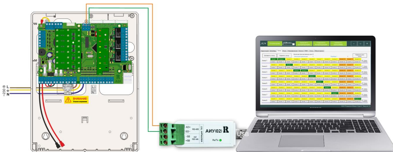
Рисунок 94. Схема подключения для конфигурирования ППКПиУ А24
