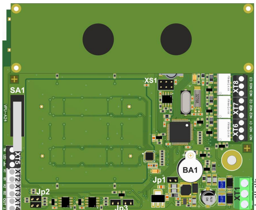
Рисунок 14. Внешний вид и обозначение элементов платы ВПУ-А24/700.
