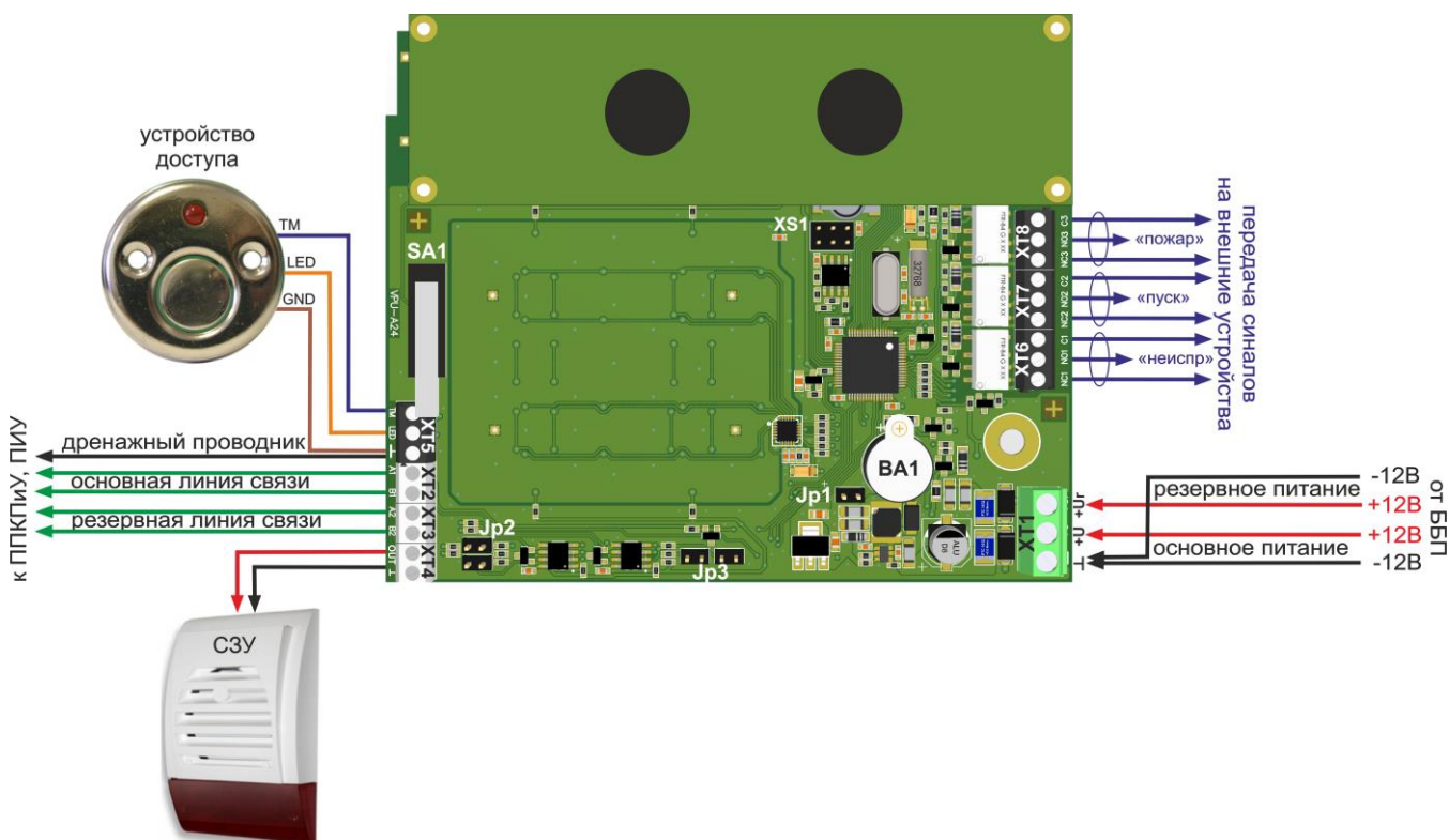
Рисунок 15. Схема подключения ВПУ-A24/700
