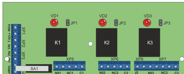
Рисунок 81. Внешний вид платы и обозначение элементов БУН3-12
