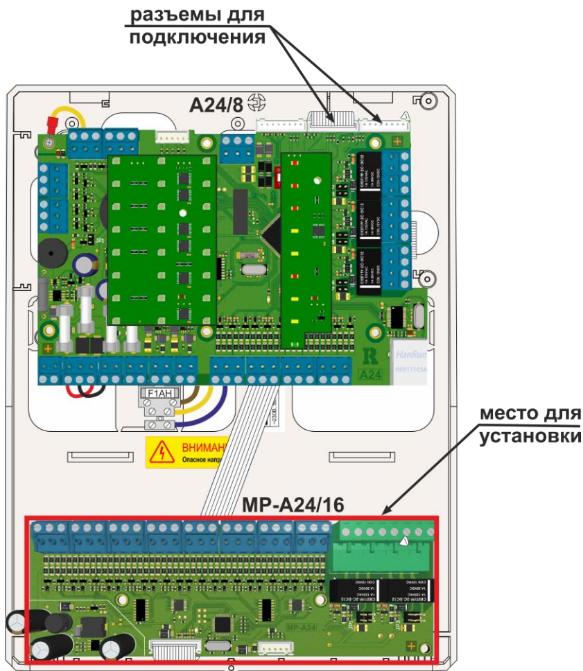
Рисунок 7. Установка и подключение MP-A24/16 к ППКПиУ
