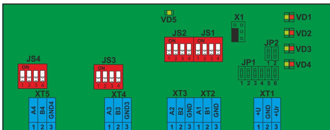
Рисунок 73. Внешний вид платы P485
