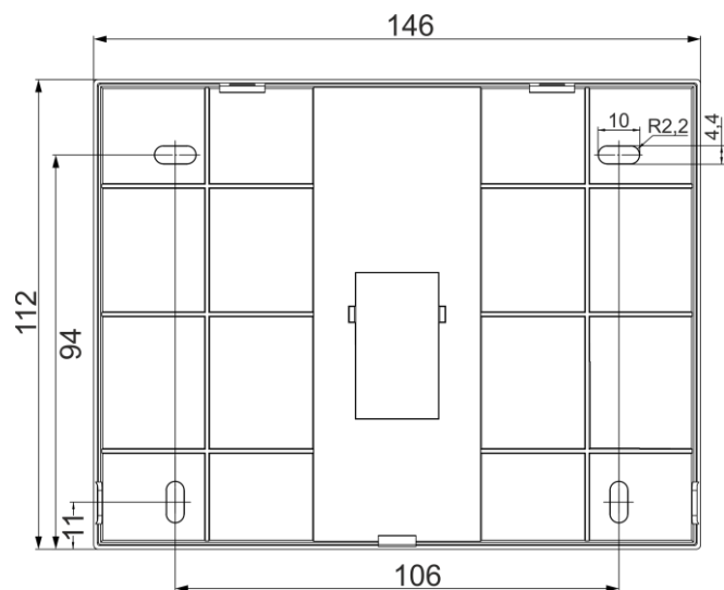
Рисунок 86. Установочный чертеж основания корпуса ВПУ-А24/700
