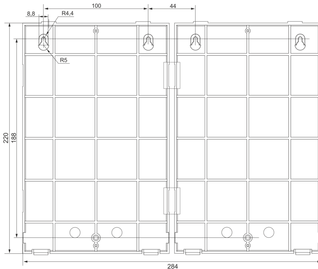
Рисунок 88. Установочный чертеж основания корпуса ПИУ-А24А и ПИУ-А24Б при применении совместно с одной ПИУ-А24Р
