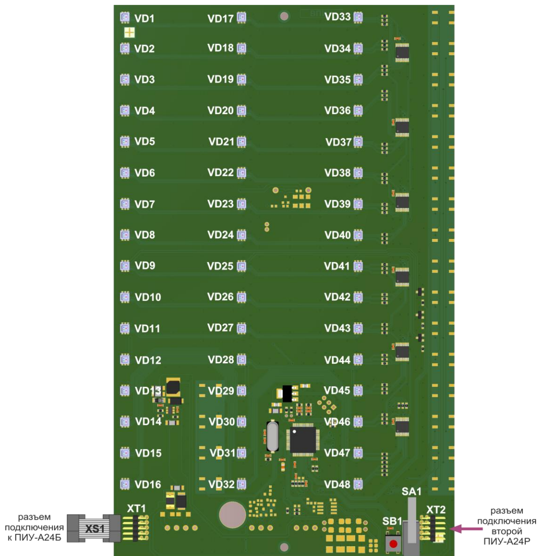
Рисунок 69. Внешний вид и подключение платы ПИУ-A24P
