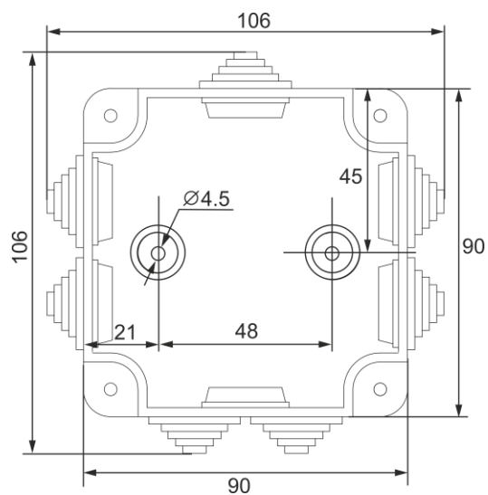
Рисунок 92. Установочный чертеж БУН1-12С
