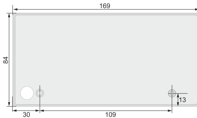
Рисунок 91. Установочный чертеж БУН3-12
