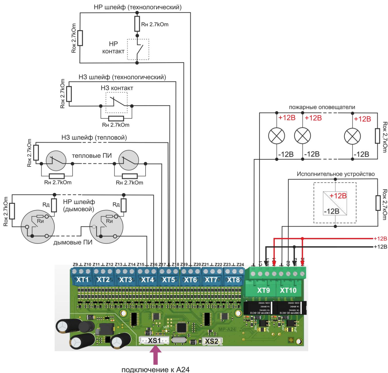
Рисунок 9. Схема подключения MP-A24/16
