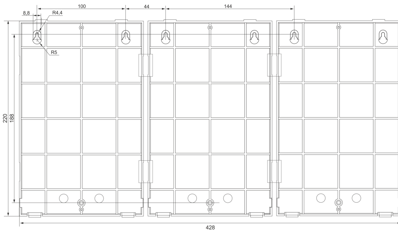
Рисунок 89. Установочный чертеж основания корпуса ПИУ-А24Б при применении совместно с двумя ПИУ-А24Р
