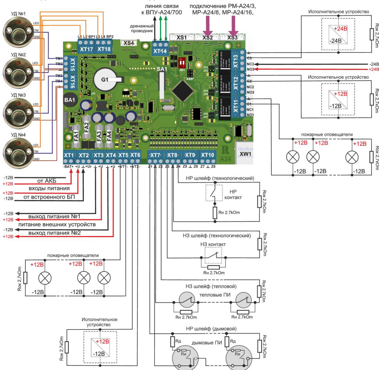
Рисунок 6. Схема подключения А24/8
