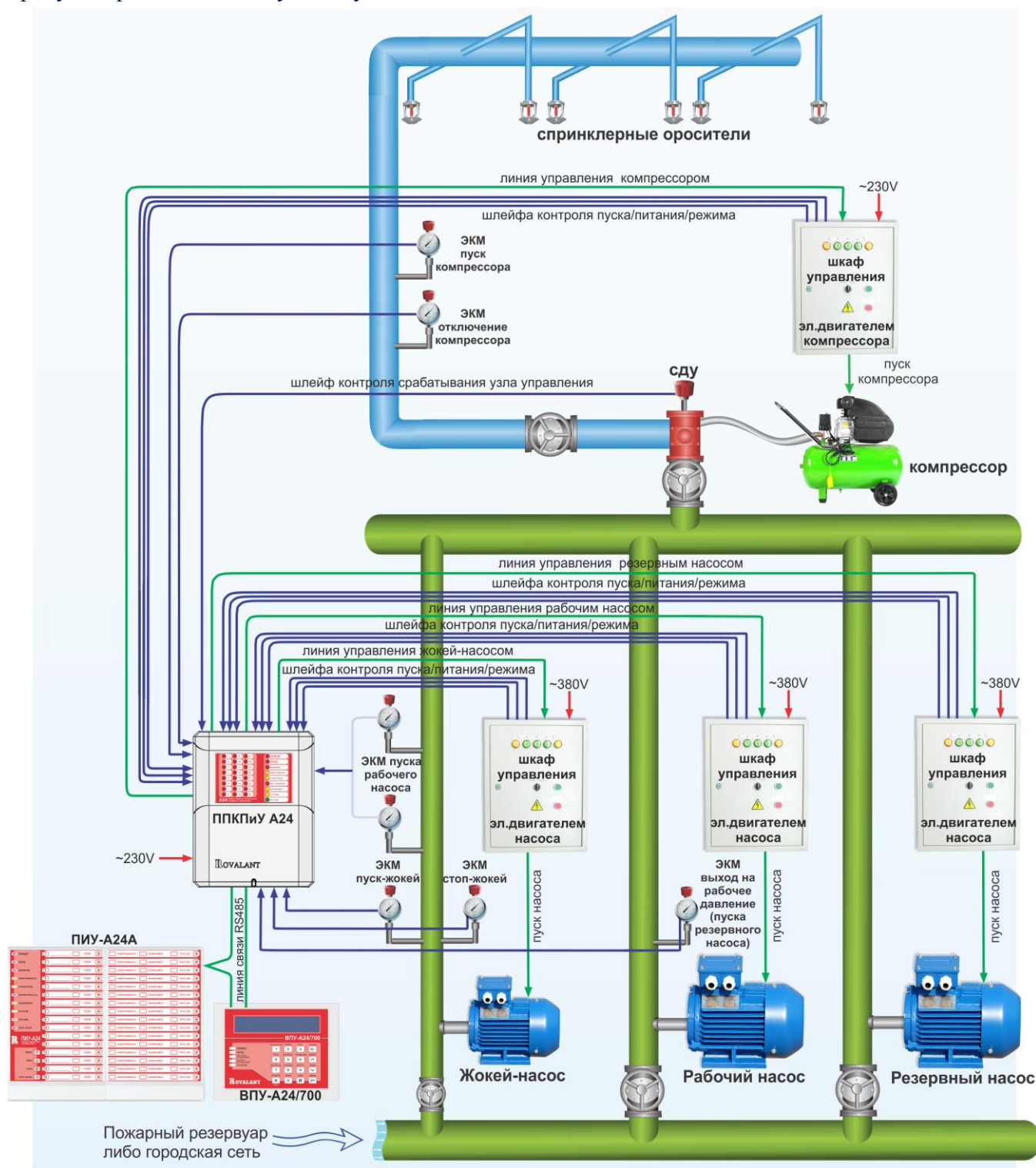
Рисунок 99. Пример автоматизации спринклерной установки воздухозаполненной системы водяного АПТ.
