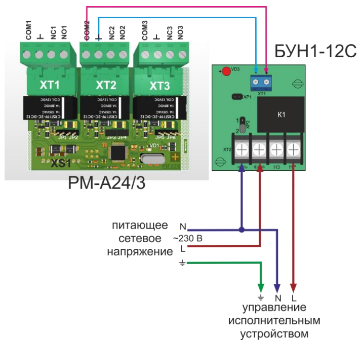
Рисунок 79. Схема подключения БУН1-12С к РМ-А24/3.
