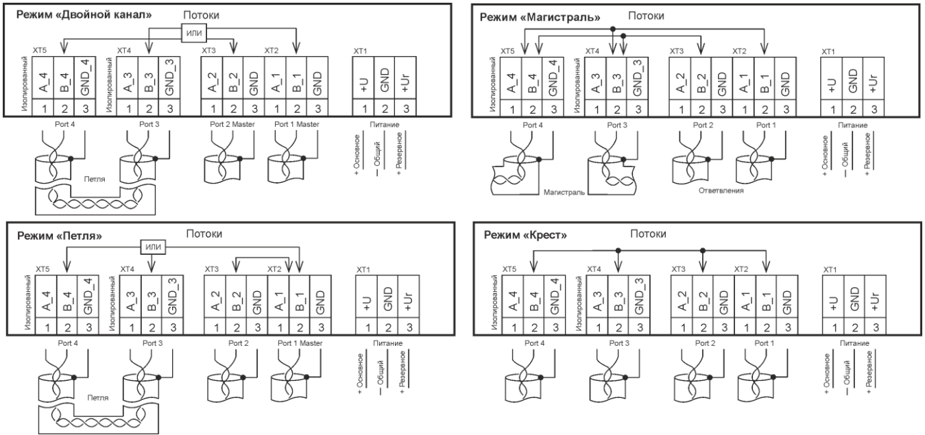
Рисунок 74. Подключение P485 при различных режимах его работы
