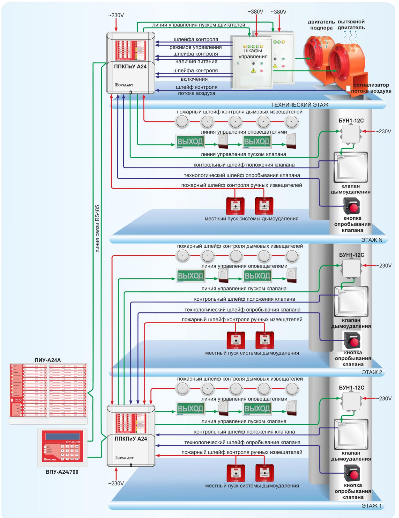
Рисунок 95. Пример структурной схемы построения систем ПС, СО и ДУ.
