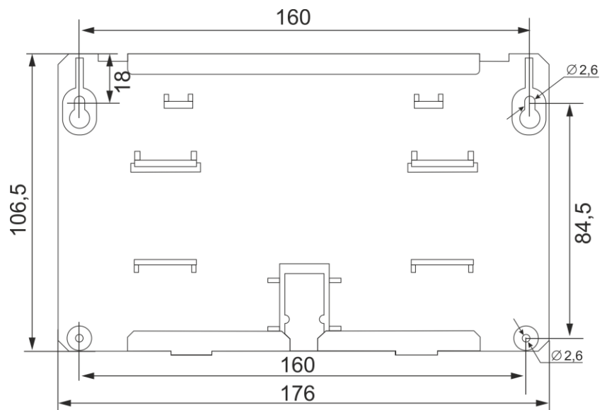
Рисунок 90. Установочный чертеж основания корпуса P485
