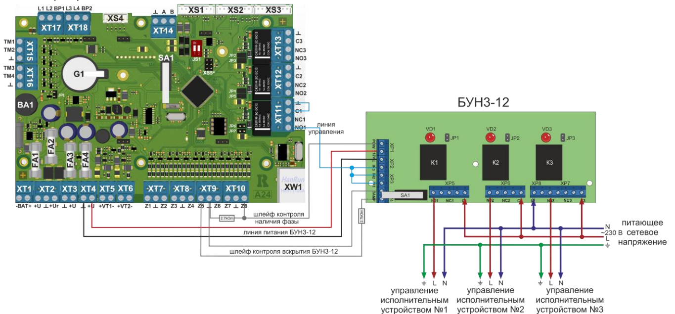
Рисунок 82. Схема подключения БУНЗ-12 к ППКПиУ А24/8.
