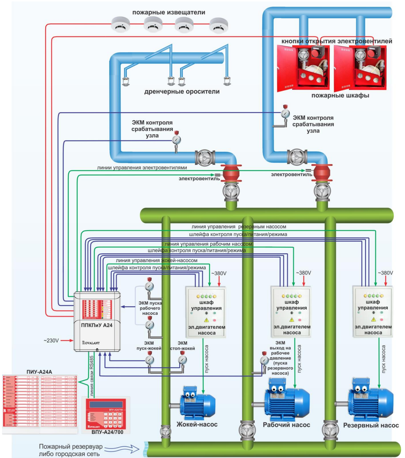
Рисунок 100. Пример автоматизации дренчерной установки системы водяного АПТ.
