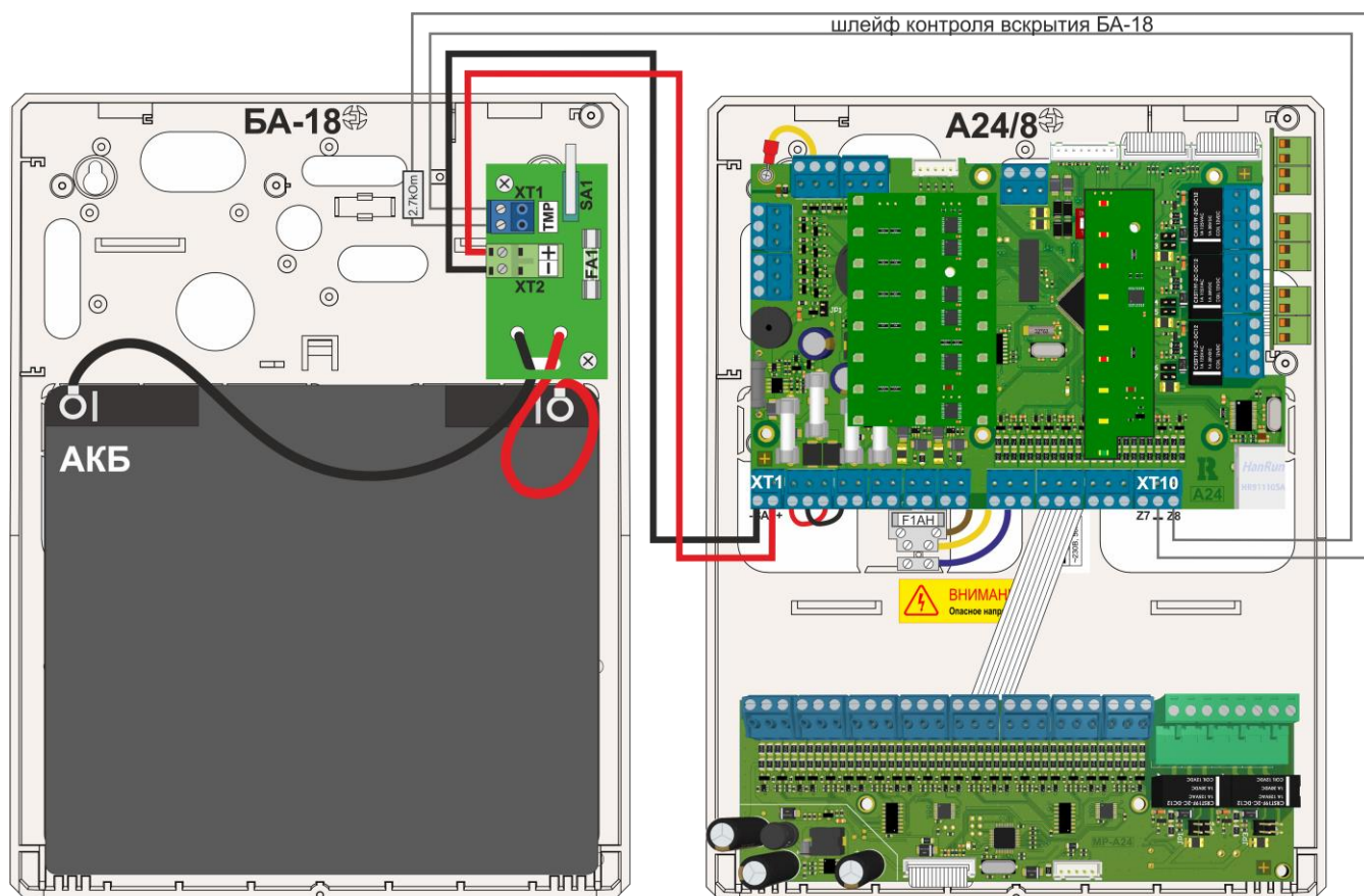
Рисунок 84. Схема подключения БА-18 к ППКПиУ А24/8.
