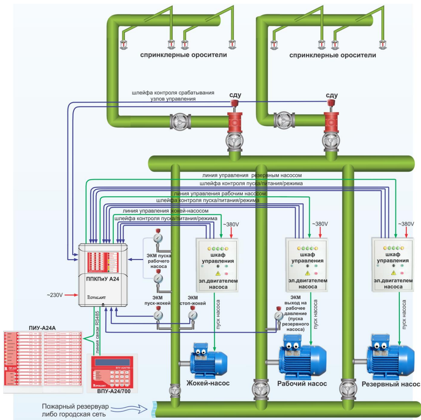
Рисунок 98. Пример автоматизации спринклерной установки водозаполненной системы водяного АПТ.
