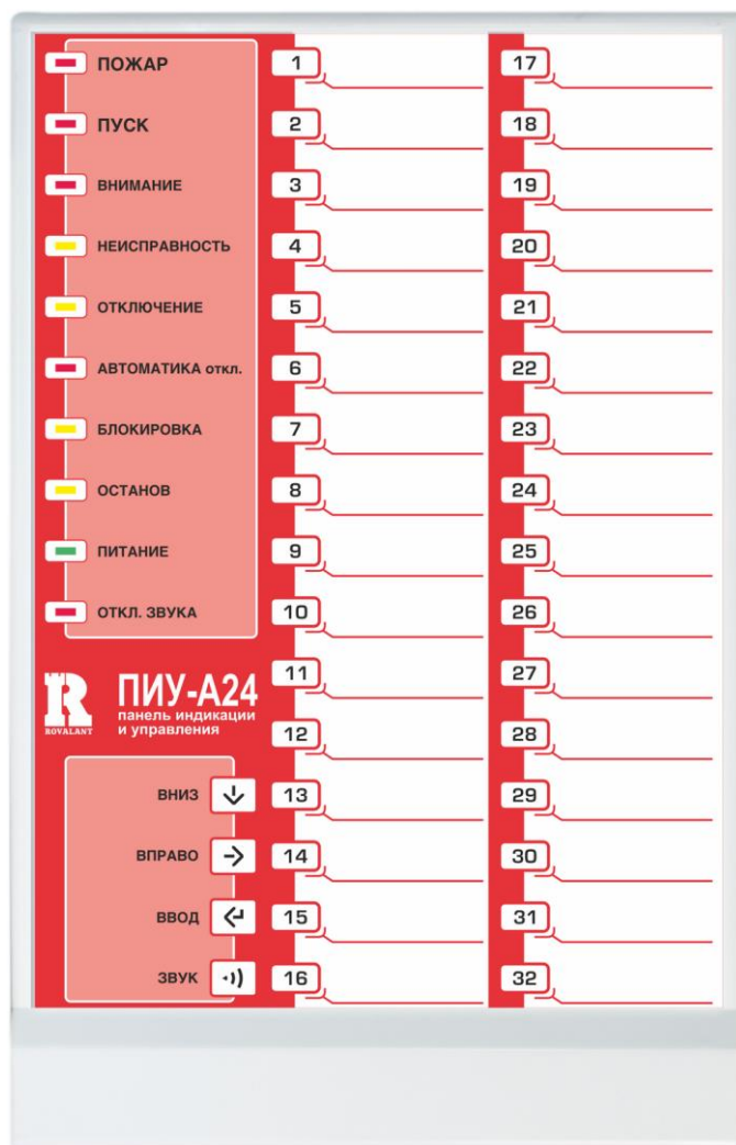
Рисунок 65. Внешний вид ПИУ-А24Б
