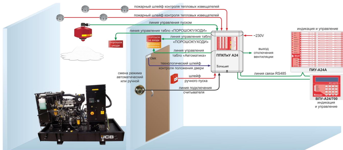
Рисунок 97. Пример автоматизации системы модульного порошкового АПТ
