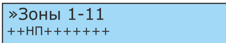
Рисунок 42. Просмотр состояния пожарных зон прибора кратко
