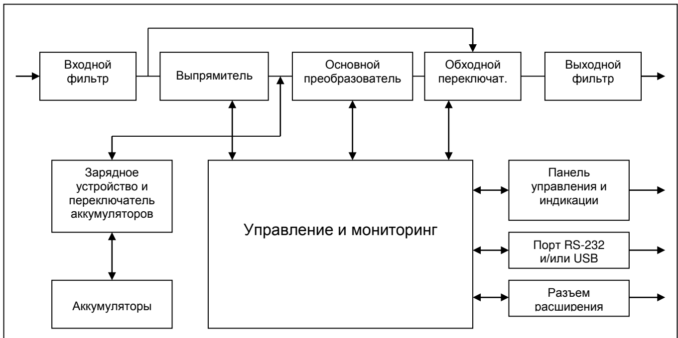
Рис. 7. Блок-схема ИБП
