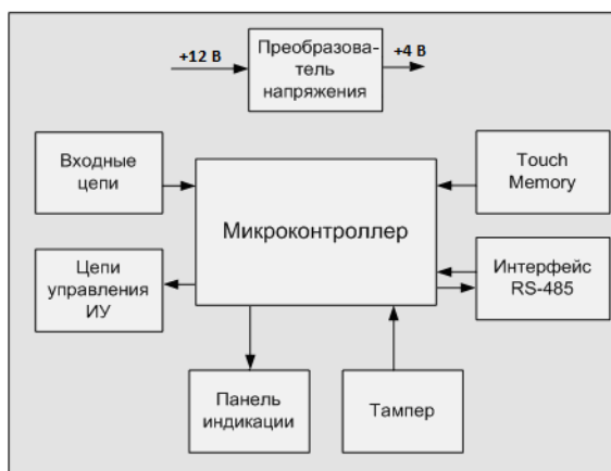
Рисунок 1.1 – Функциональная схема
