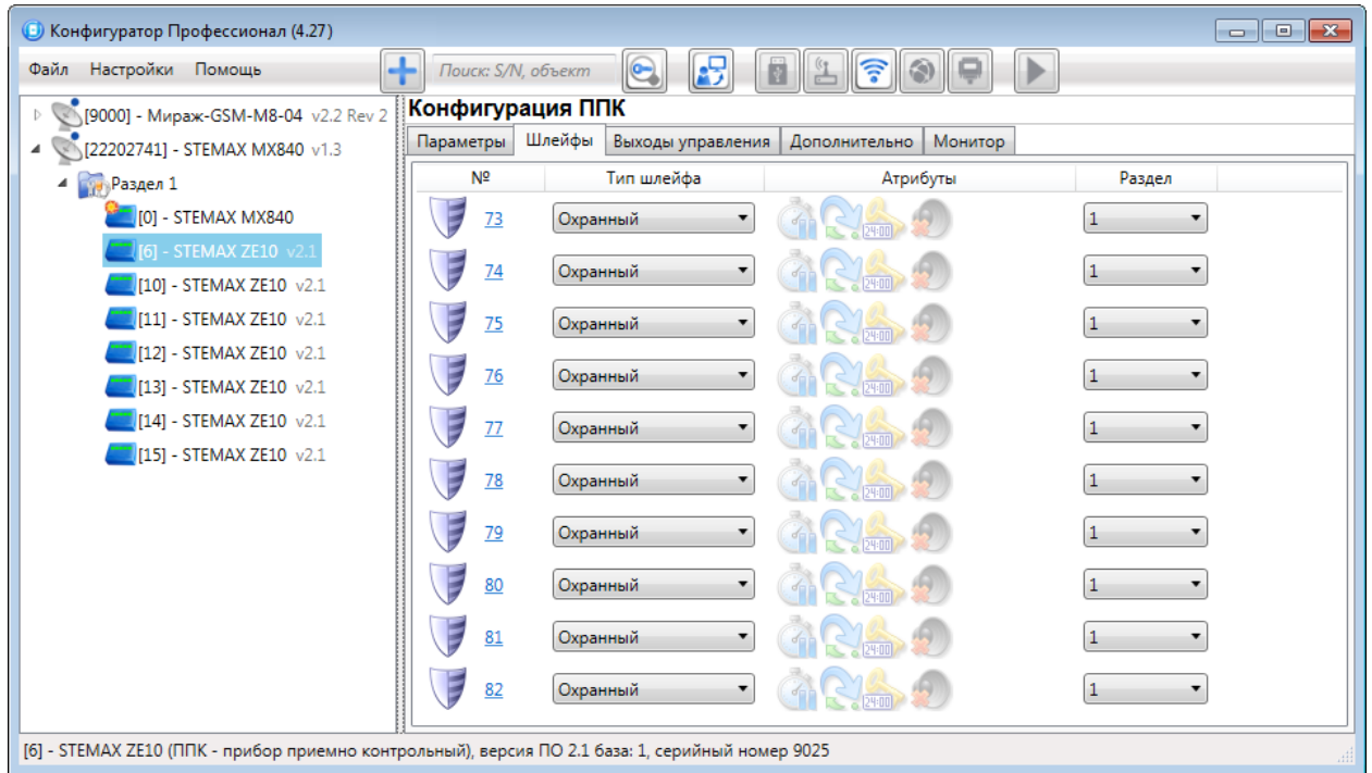
Рисунок 4.7 – Конфигурация СКП, вкладка Шлейфы
