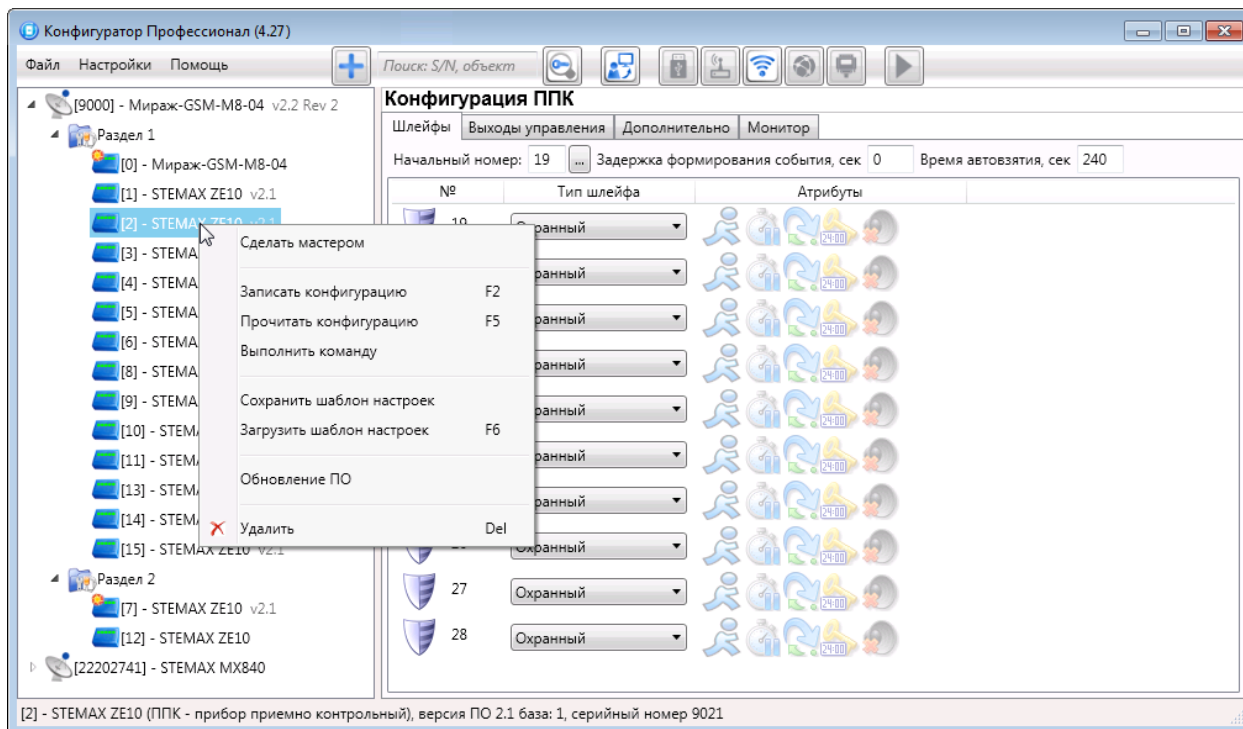
Рисунок 5.14 – Контекстное меню панели
