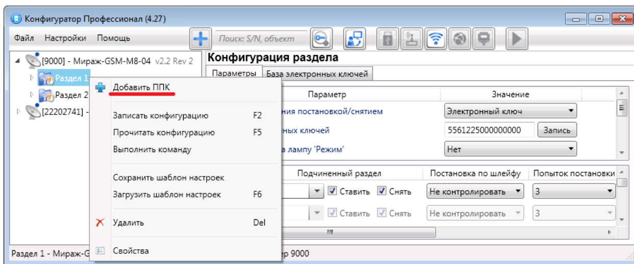
Рисунок 5.1 — Добавление панели в существующий раздел
