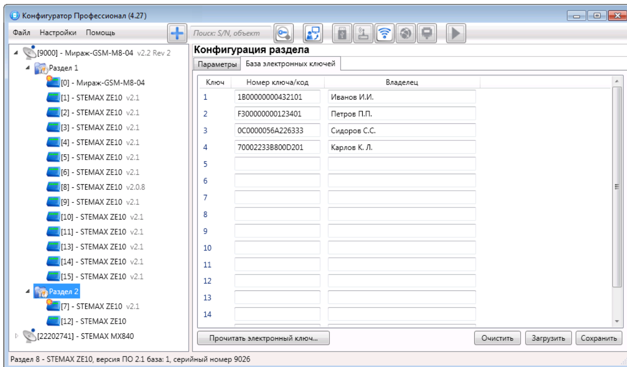
Рисунок 5.12 – Вкладка База электронных ключей
