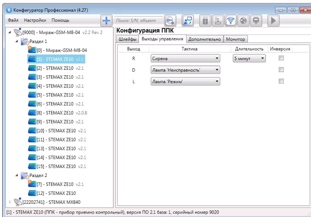
Рисунок 5.8 – Вкладка Выходы управления
