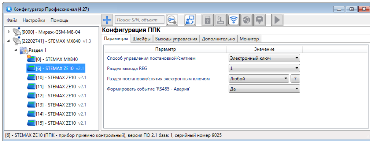
Рисунок 4.3 – Конфигурация СКП, вкладка Параметры
