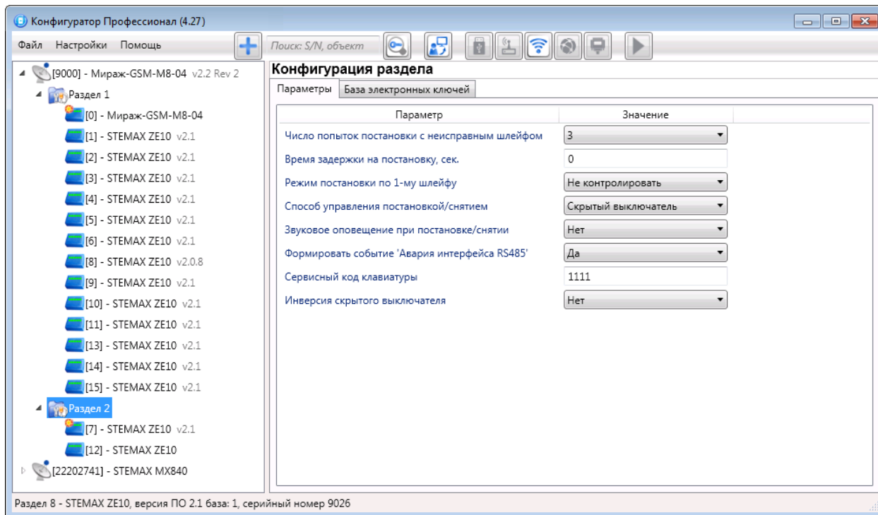
Рисунок 5.11 – Конфигурация раздела, вкладка Параметры
