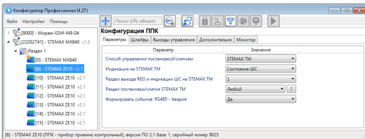
Рисунок 4.5 – Конфигурация СКП, вкладка Параметры
