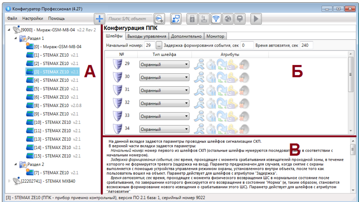
Рисунок 3.4 — Структура основного окна программы (А — дерево устройств, Б — область параметров, В — область подсказок)
