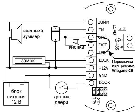
Рис.3 Подключение устройств
