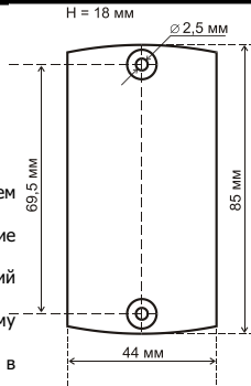
Рис.2 Габаритные размеры
