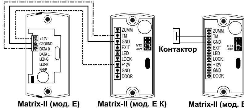
Рис. 4 Подключение внешнего считывателя
