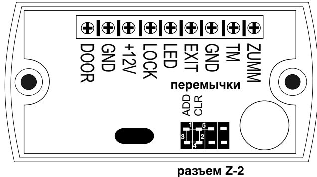
Рис. 3 Положение перемычек
