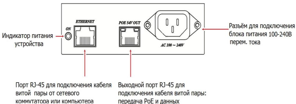
Рис.3 Разъёмы инжектора IP061.
