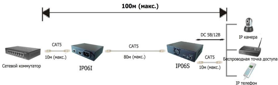
Рис.2 Схема подключения инжектора IP061 и сплиттера IP06S.
