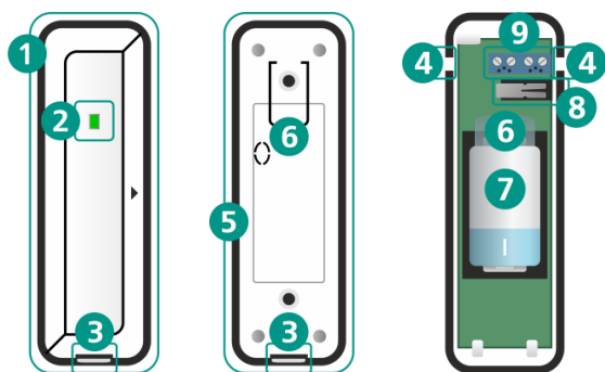
Рисунок 2.18 – Внешний вид универсального датчика
