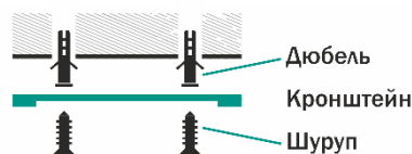
Рисунок 5.2 – Монтаж кронштейна крепления к потолку
