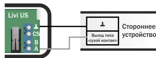
Рисунок 5.9 – Схема подключения одного устройства к датчику
