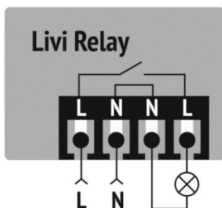
Рисунок 4.14 – Схема подключения силового реле
