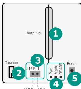
Рисунок 2.15 – Схема подключений ретранслятора
