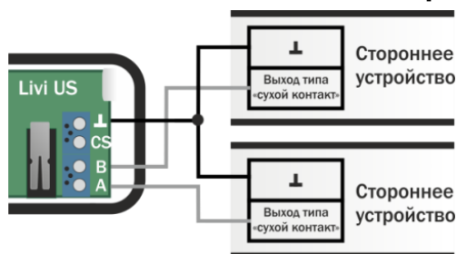
Рисунок 5.8 – Схема подключения двух устройств к датчику
