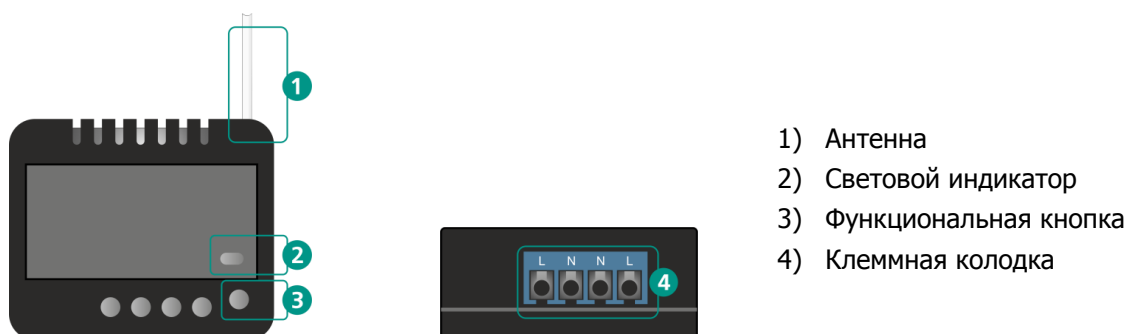
Рисунок 2.12 – Внешний вид реле Livi Relay и Livi Relay 12/24
