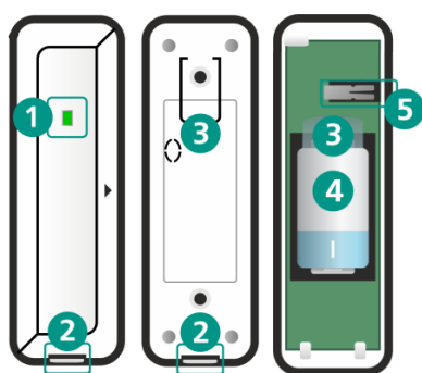
Рисунок 2.9 – Внешний вид датчика удара
