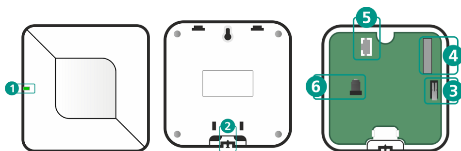
Рисунок 2.13 – Внешний вид ретранслятора Livi RTRM
